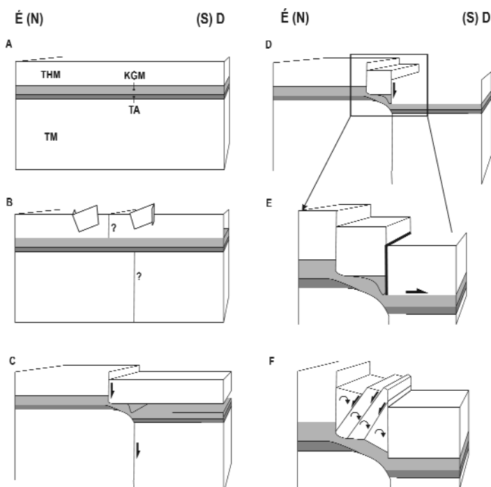
5. ábra. A Tölgyhát-kőfejtő keleti feltárásában található szerkezet kialakulásának nem méretarányos modellje Magyarázat a szövegben
