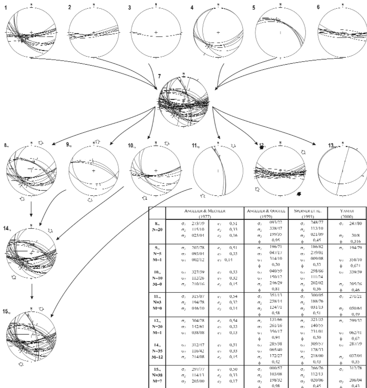
4. ábra. A Tölglyhát-kőfejtőben talált vetőkarc-csoportok Schmidt-félgömbön, alsó vetítés
