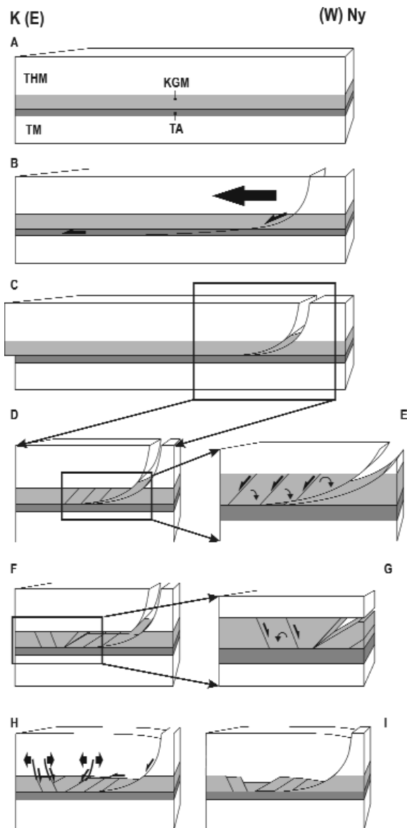
6. ábra. A Tölgyhíti-kőfejtő nyugati feltárásában található szerkezet kialakulásának nem méretarányos modellje Magyarázat a szövegben
